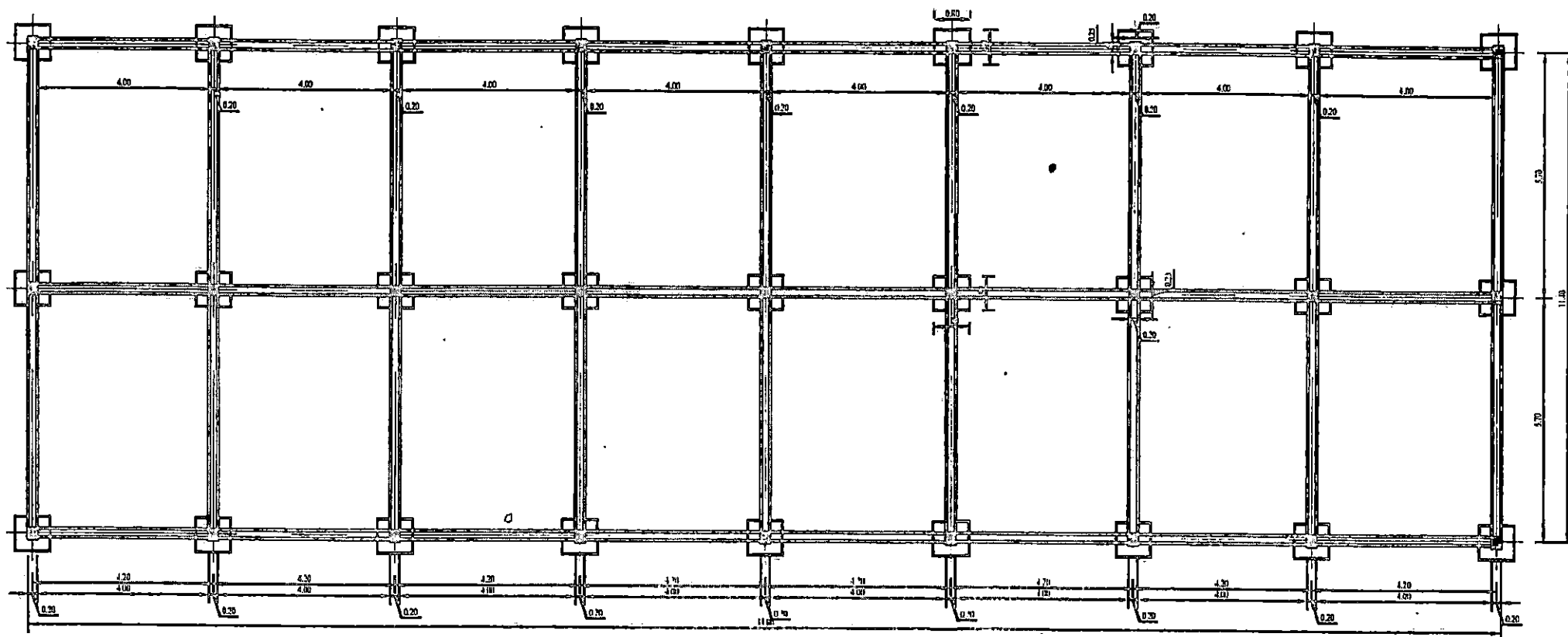
PLAN DE FONDATION ATELIER MENUISERIE
